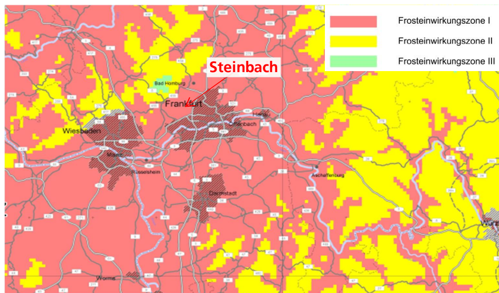
Abbildung 7: RStO Frostwirkungszone (Ausschnitt)
